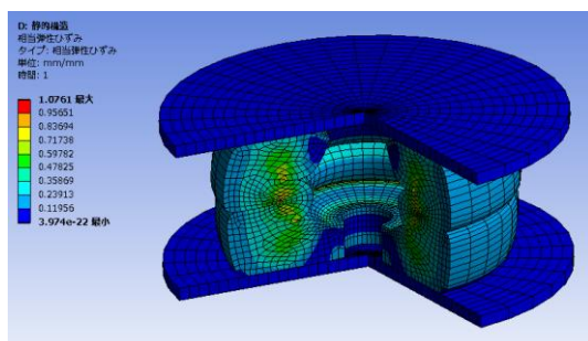
提灯型クッションのCAE解析結果
