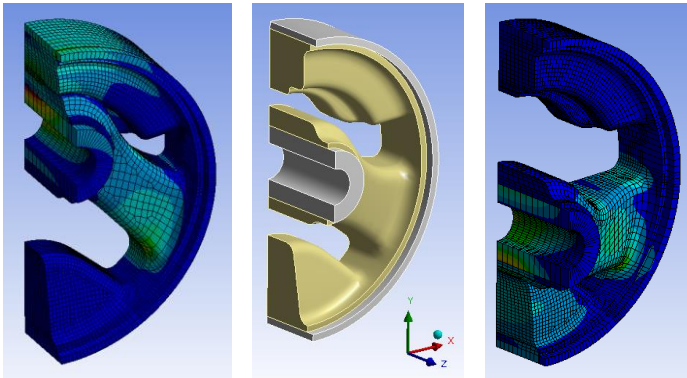
八の字型マウントのCAE解析結果
